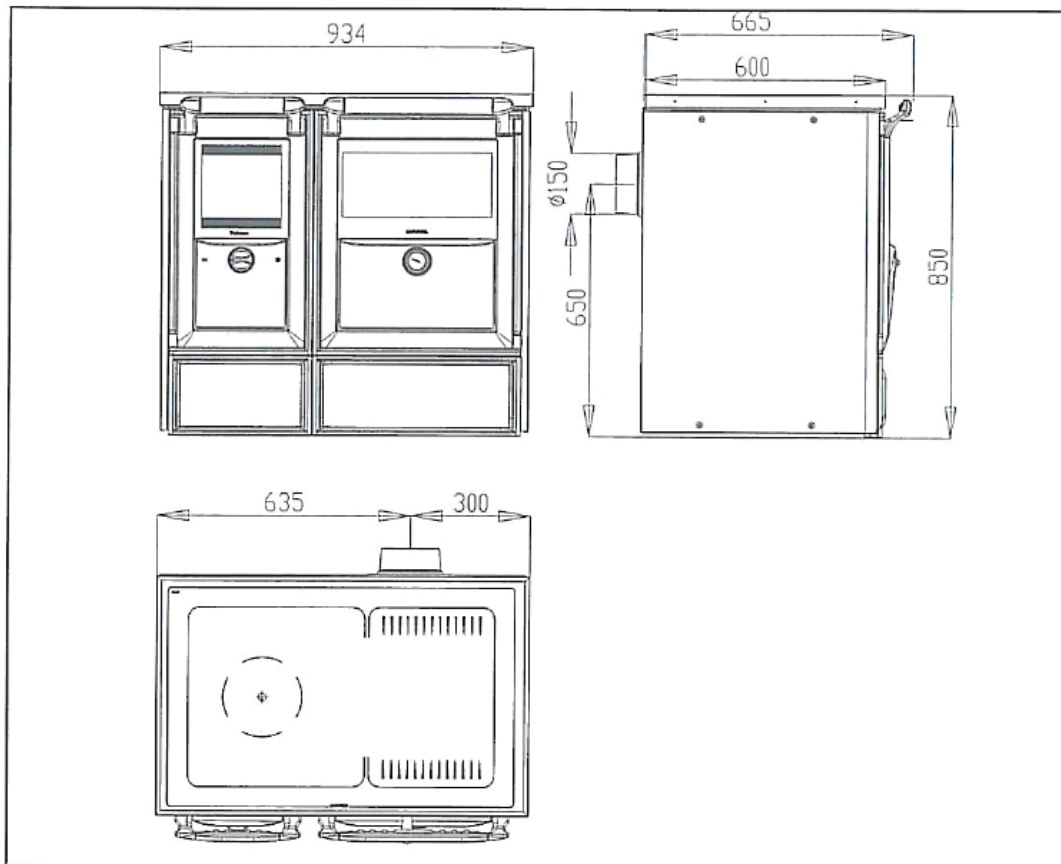
Figura n°3 – Dimensiones en mm Cocina Vulcano 7.
