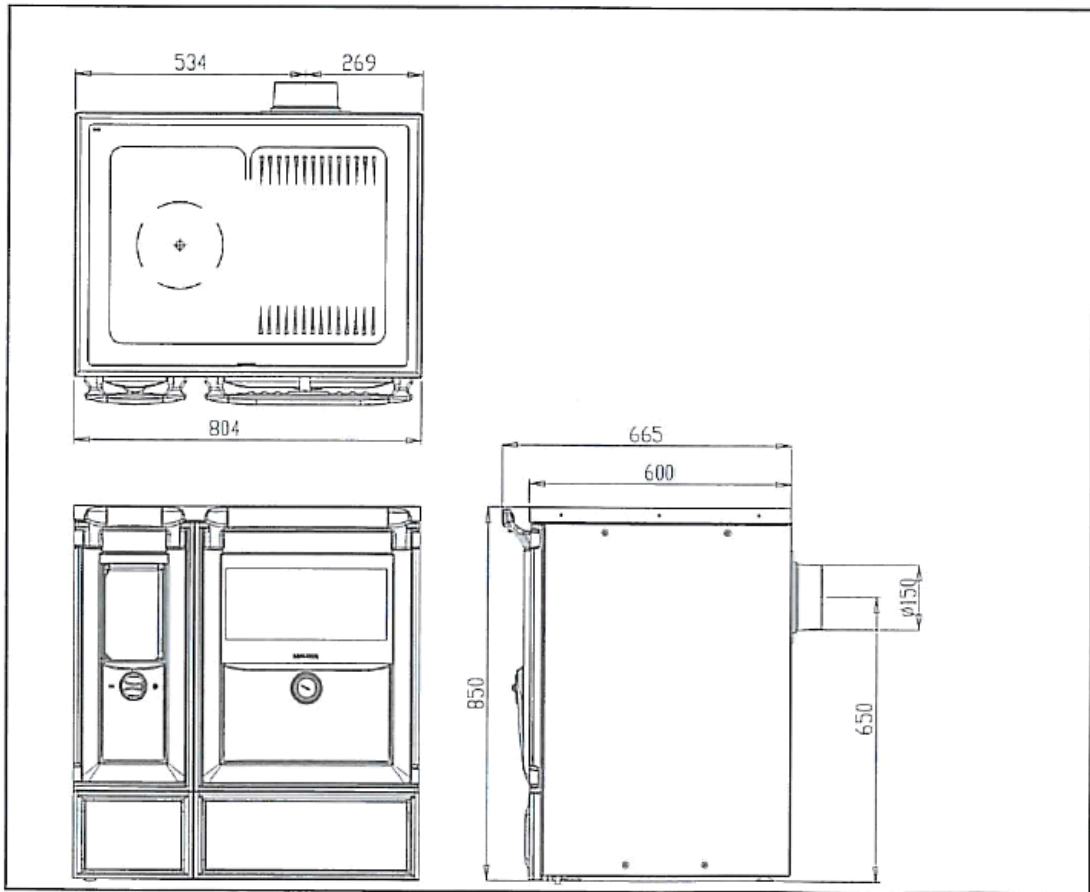
Figura n°2 – Dimensiones en mm Cocina Vulcano 5.
